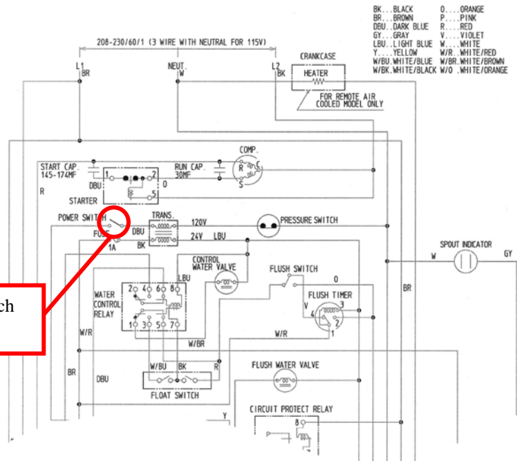
New Wiring
